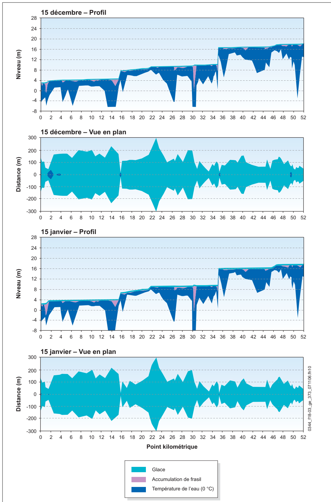
Figure 18-3 : Emprise de la couverture de glace en aval de la centrale de la Romaine-1 – Hiver de rigueur moyenne (15 décembre et 15 janvier) – Conditions actuelles
