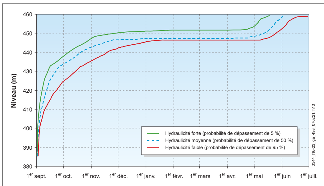
Figure 16-23 : Courbe de remplissage du réservoir de la Romaine 4 selon l'hydraullicité
