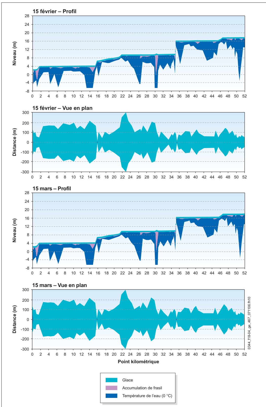
Figure 18-4 : Emprise de la couverture de glace en aval de la centrale de la Romaine-1 – Hiver de rigueur moyenne (15 février et 15 mars) – Conditions actuelles
