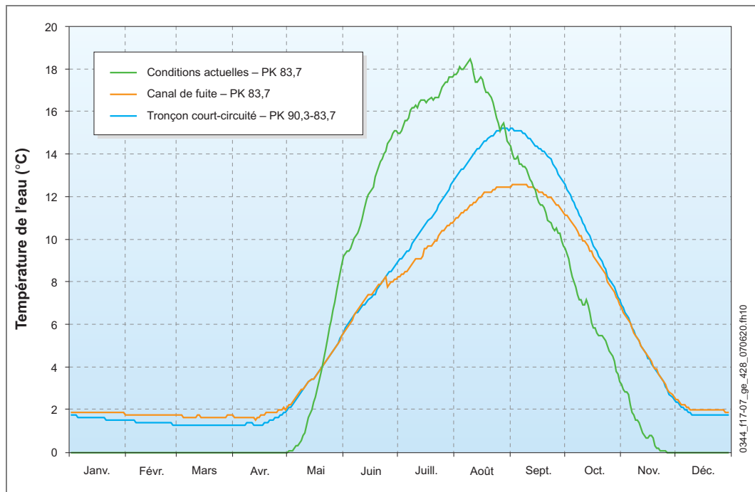
Figure 17-7 : Température de l'eau au PK 83,7 de la Romaine (canal de fuite de la Romaine-2) – Conditions actuelles et futures
