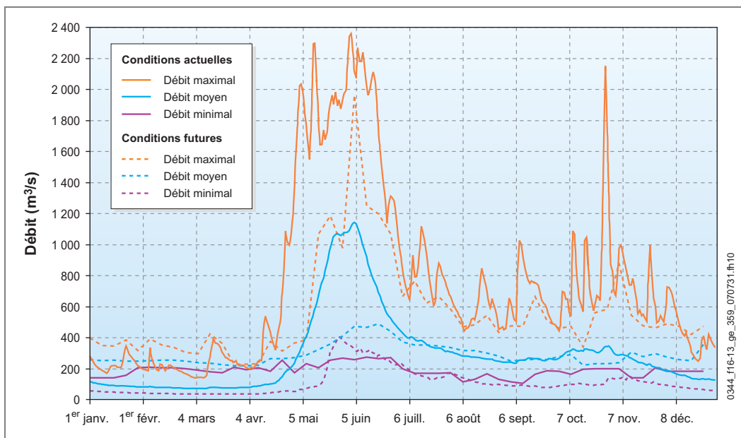
Figure 16-13 : Débits totaux hebdomadaires (turbinés et déversés) au site de la Romaine-1 – Conditions actuelles et futures
